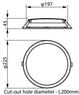
DN065B G3 LDNR LED20/830 19.5W D200 RD
