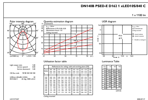
IFGU1_DN140BPSED-ED1621xLED10S840C
