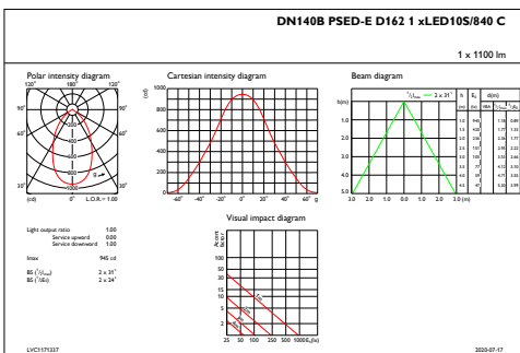
IFAS1_DN140BPSED-ED1621xLED10S840C
